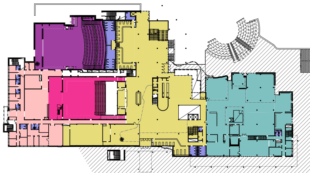
TILATYYPIT 1. kerros 1:1000
