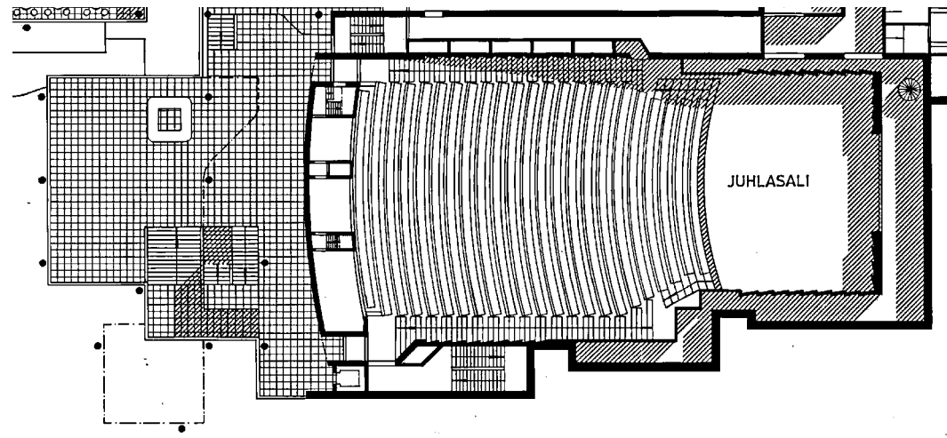
↓ 2.krs pohjapiirros, ote juhlasalin kohdalta Juhlasali permanto, kuvassa vasemmalla salin päälämpiö. Esittelypohjapiirros vuodelta 1989, Arkkitehtitoimisto Arto Sipinen Ky. ASA
